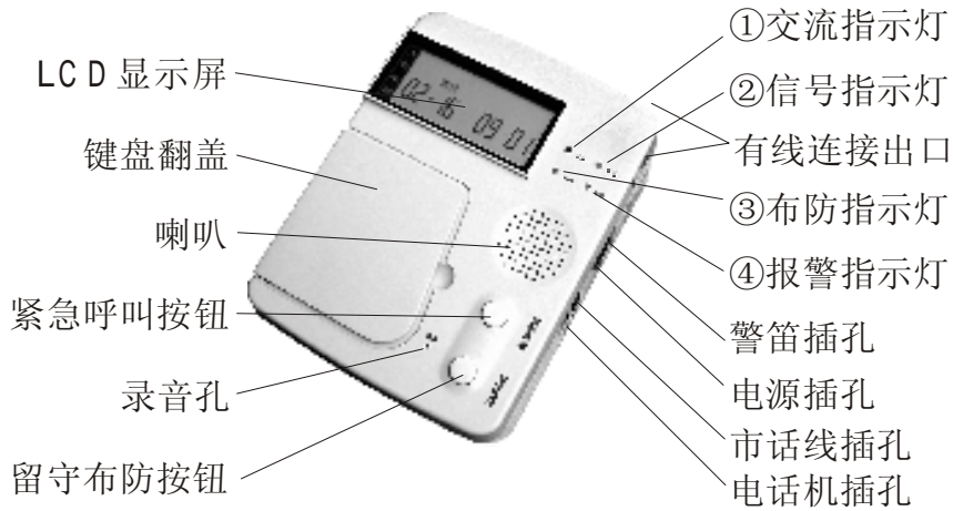
主机正面结构示意图
